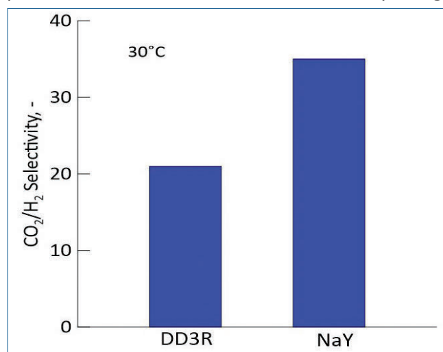
Fig. 4 - Selettività \text{CO}_2/\text{H}_2 per una miscela equimolare a 30 °C in NaY e DD3R
