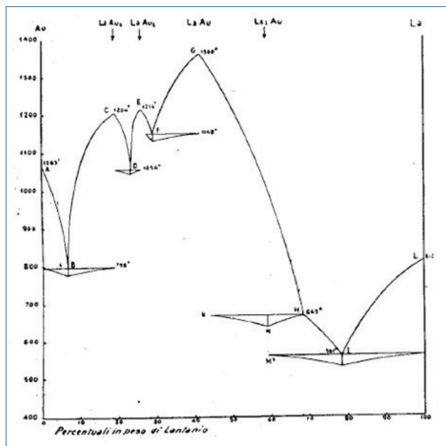
Fig. 2 - Diagramma di stato della lega lantanio oro, immagine tratta da La metallurgia italiana , 1931, 23, 818
