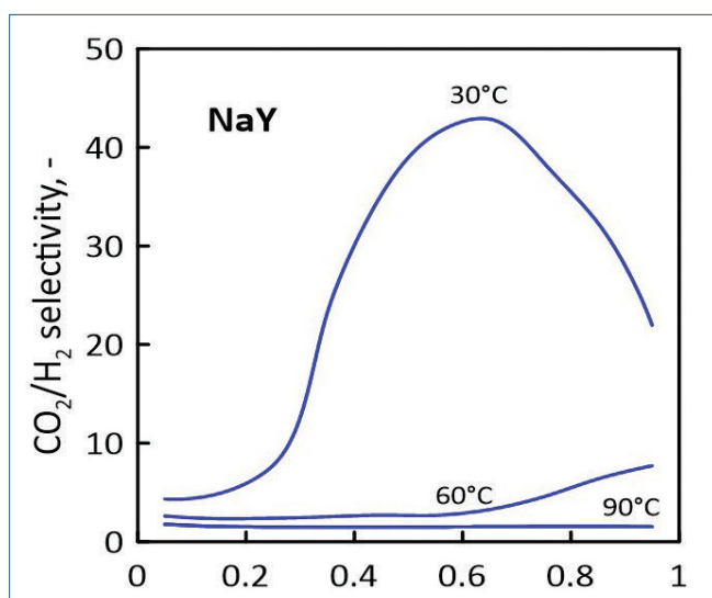
Fig. 3 - Selettività di \text{CO}_2/\text{H}_2 al variare della composizione di alimentazione a diverse temperature in NaY
