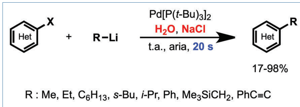
Fig. 1 - Reazione di tipo Muharashi palladio catalizzata "on water"
