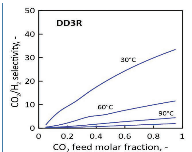
Fig. 2 - Selettività di \text{CO}_2/\text{H}_2 al variare della composizione di alimentazione a diverse temperature in DD3R
